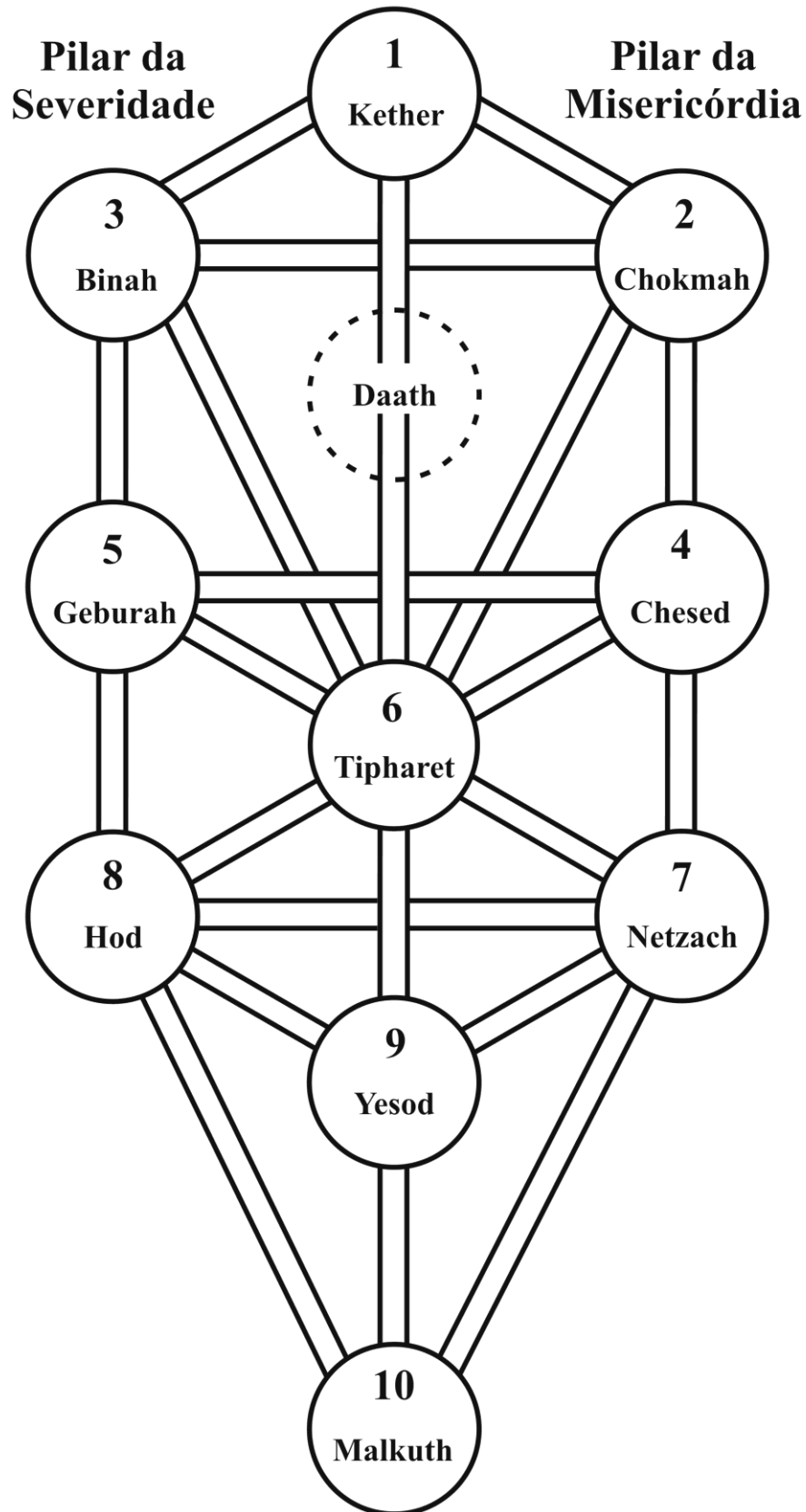
Disposição das Sephiroth na Árvore da Vida
