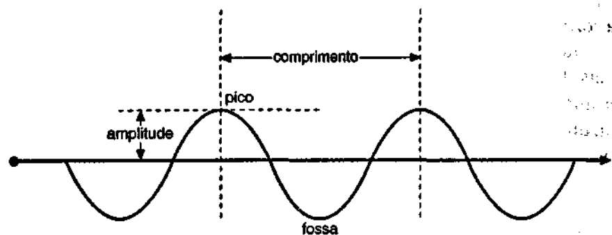
Figura 4. Representação gráfica de uma onda.
