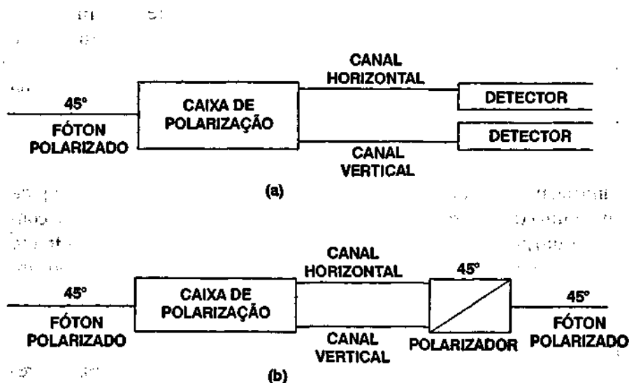
Figura 28. Experimentos com fótons polarizados a 45°.
