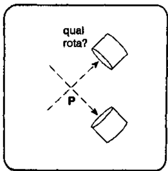
Figura 20. O experimento de escolha retardada. CANTO INFERIOR ESQUERDO: o arranjo para ver a natureza de onda do elétron. Um dos detectores jamais detecta quaisquer fótons, significando isto cancelamento devido à interferência de onda. O fóton deve ser dividido e viajado por ambas as rotas na mesma ocasião. CANTO INFERIOR DIREITO: arranjo para ver a natureza de partícula do fóton. Ambos os detectores clicam – embora apenas um de cada vez – indicando qual a rota tomada pelo fóton.
