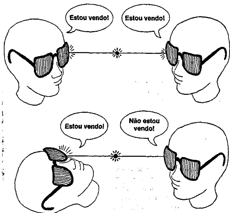
Figura 30. Observações de fótons correlacionados por polarização.
