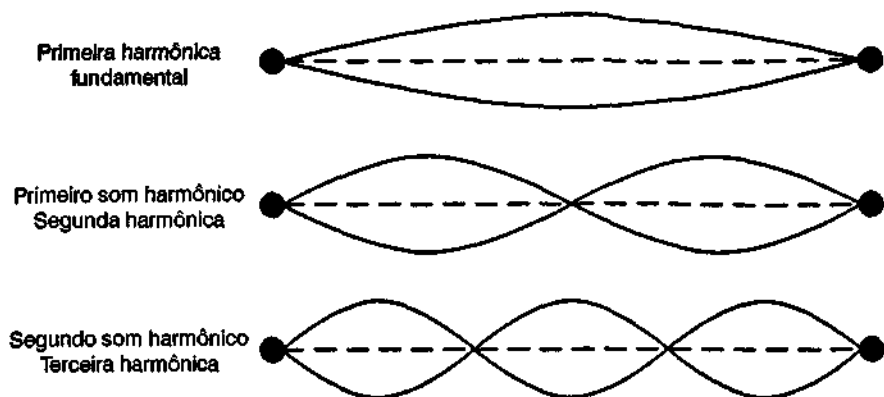
Figura 5. As primeiras harmônicas de uma onda imóvel ou estacionária em uma corda de violão.
