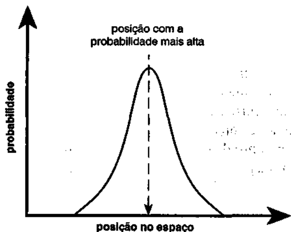
Figura 9. Uma distribuição típica de probabilidade.
