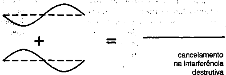
Figura 15. (a) Quando ondas de água interferem entre si, elas ocasionam um interessante padrão de reforços e cancelamentos. (b) Quando as ondas chegam em fase, elas se reforçam reciprocamente. (c) Ondas fora de fase. Resultado: cancelamento.
