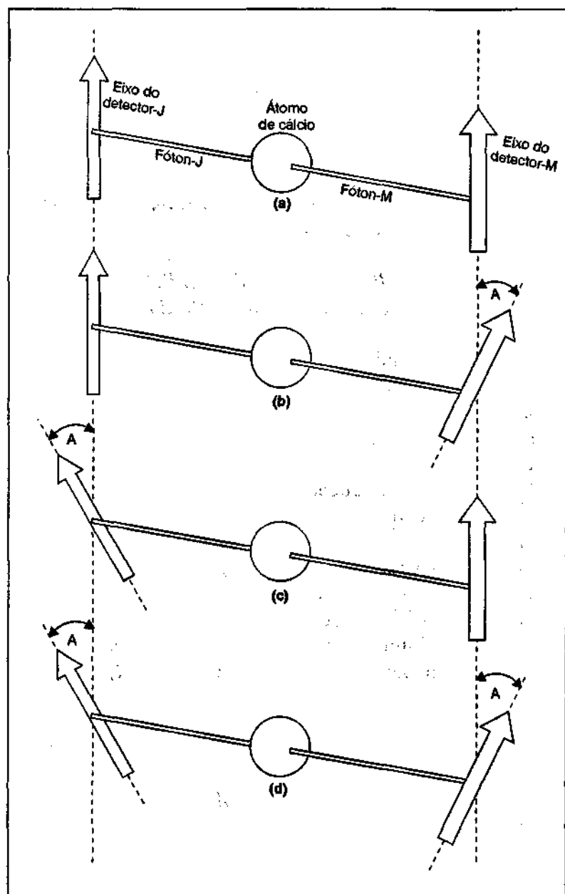
Figura 31. Maneira como surge uma desigualdade de Bell. Se as variáveis ocultas são locais, a taxa de erro (o desvio da correlação perfeita) no arranjo (d) deveria ser, no máximo, a soma das taxas de erro dos dois arranjos mostrados em (b) e (c).
