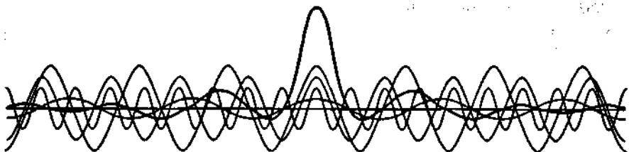
Figura 8. A superposição de ondas simples produz um pacote simples localizado de ondas. (Adaptado com permissão de P. W. Atkins, Quanta: A Handbook of Concepts . Oxford: Clarendon Press, 1974.)
