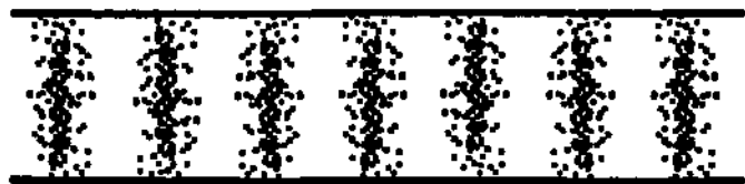
Figura 16. O padrão de interferência de lampejos na tela.
